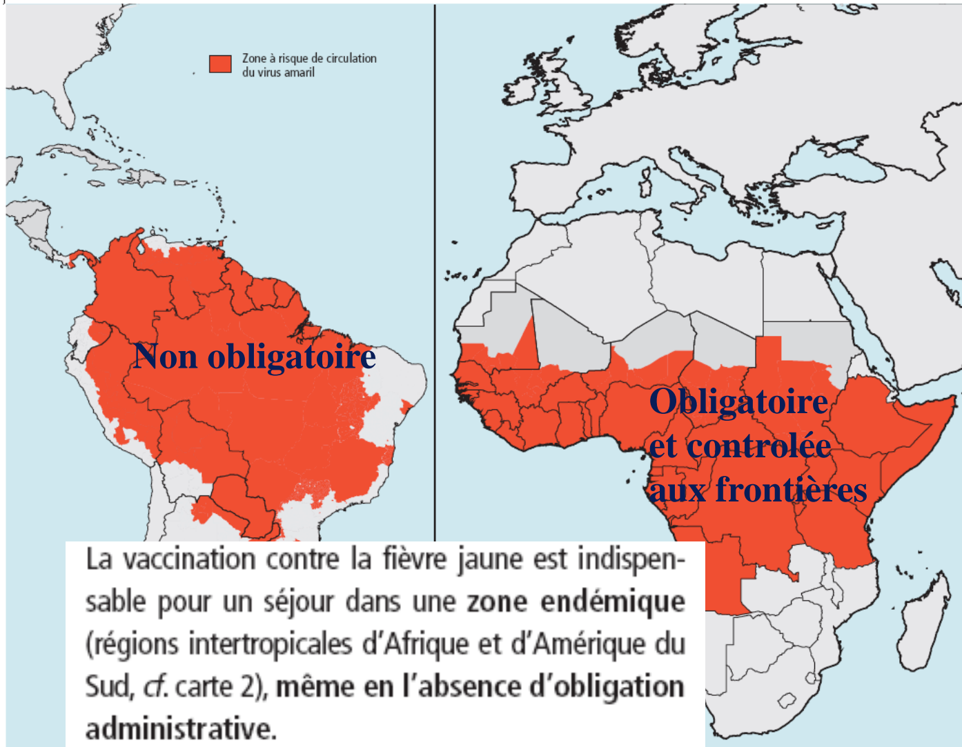
Carte 2 Zones d'endémie de la fièvre jaune
